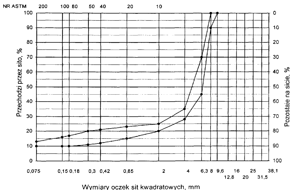
Rys. 1. Krzywe graniczne uziarnienia mieszanek mineralnej SMA od 0 do 8 mm do warstwy ścieralnej nawierzchni drogi o obciążeniu ruchem od KR3 do KR6
